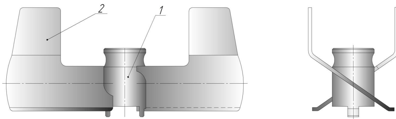
Рисунок 15 – Ротор лопастной
