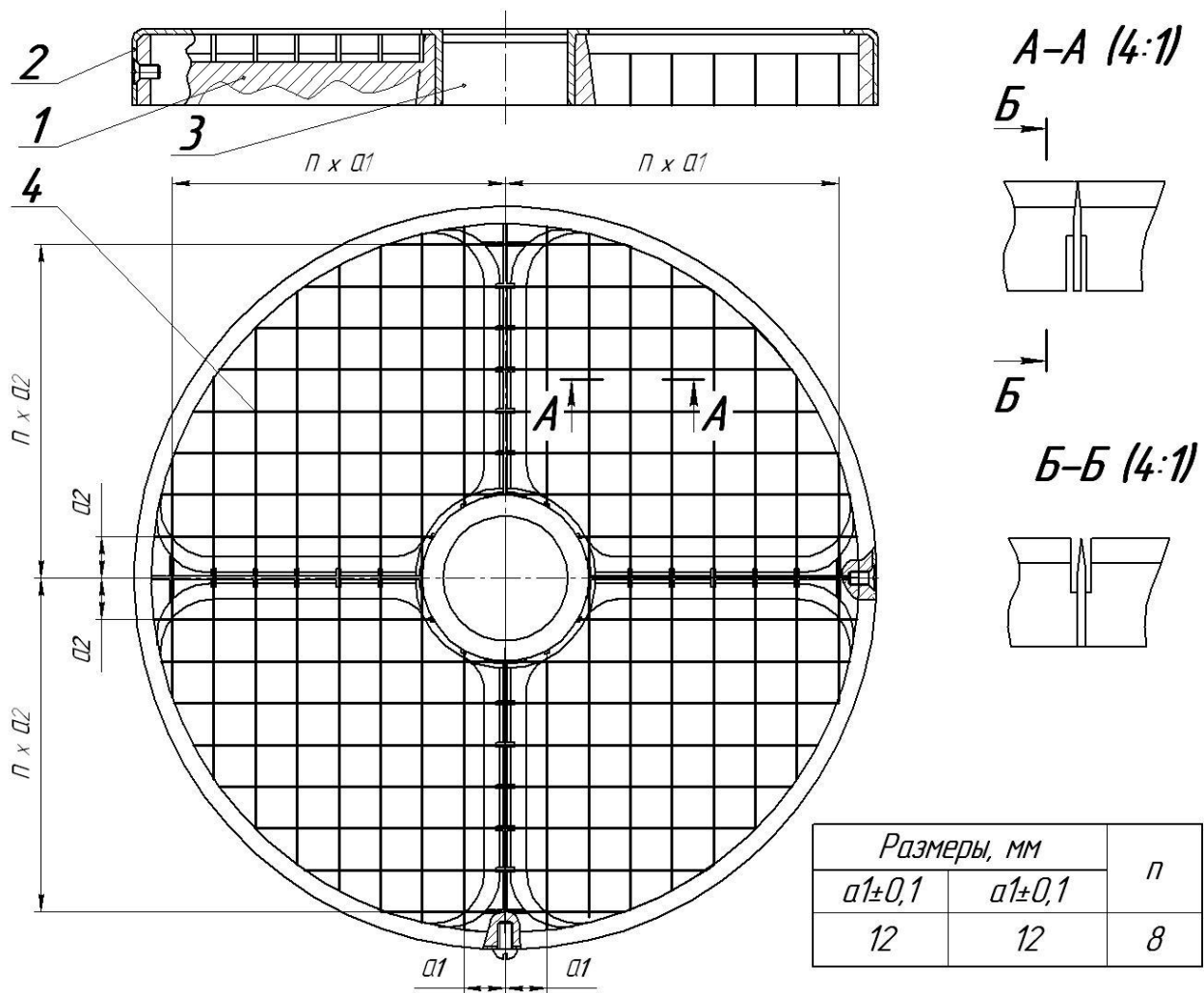
Рисунок 14 – Ножевая решетка
